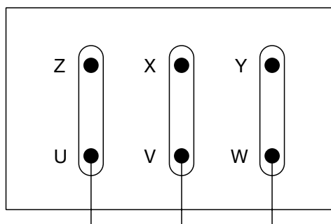
CONEXIÓN ELECTRICA EN TRIANGULO
