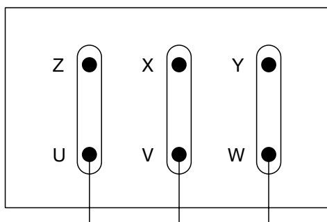
CONNEXION ÉLECTRIQUE EN TRIANGLE
